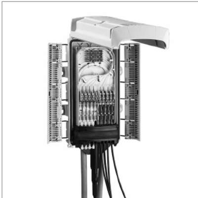
Version A: connectique LC + FAST DROP
